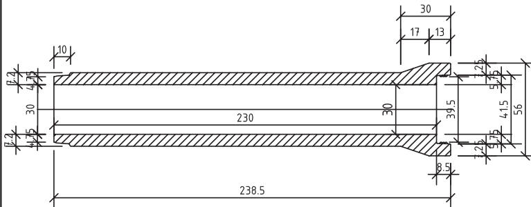
SECȚIUNE A-A
