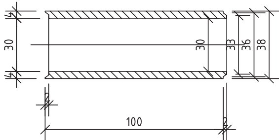
SECȚIUNE A-A
