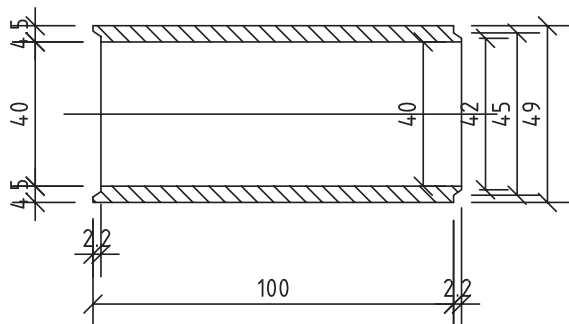
SECȚIUNE A-A
