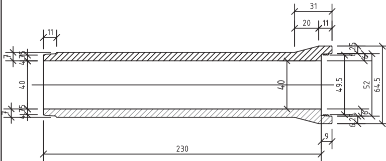
SECȚIUNE A-A
