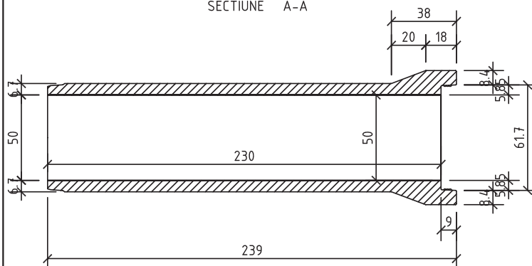
SECȚIUNE A-A
