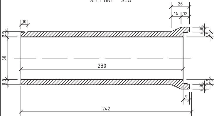
SECȚIUNE A-A
