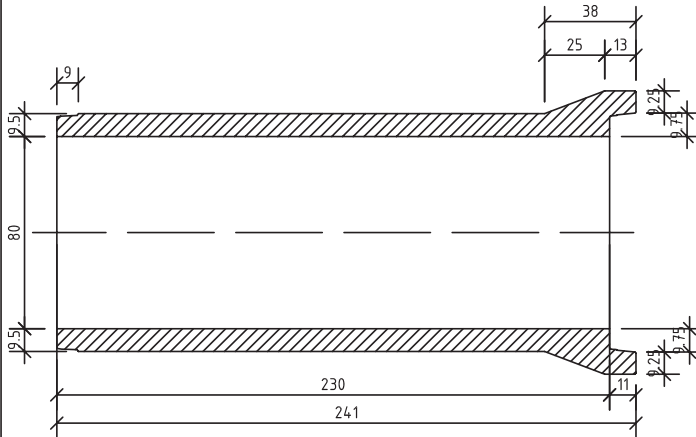
SECȚIUNE A-A
